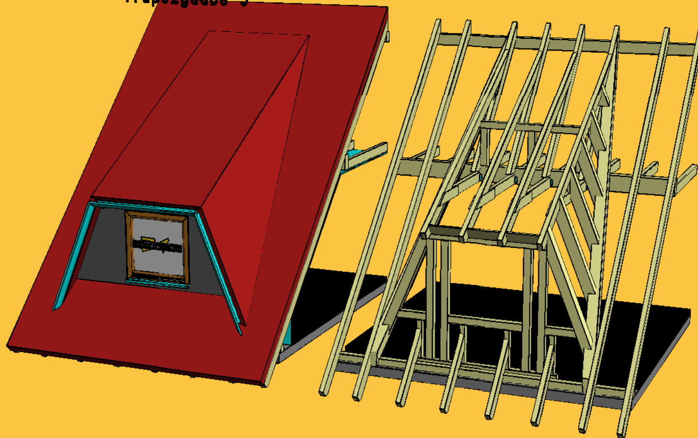
Trapezgaube 3
